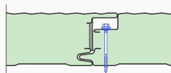
HI-PIR STM junta de panel
