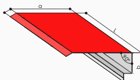
CORONACIÓN EN LATERAL DE PENDIENTE
