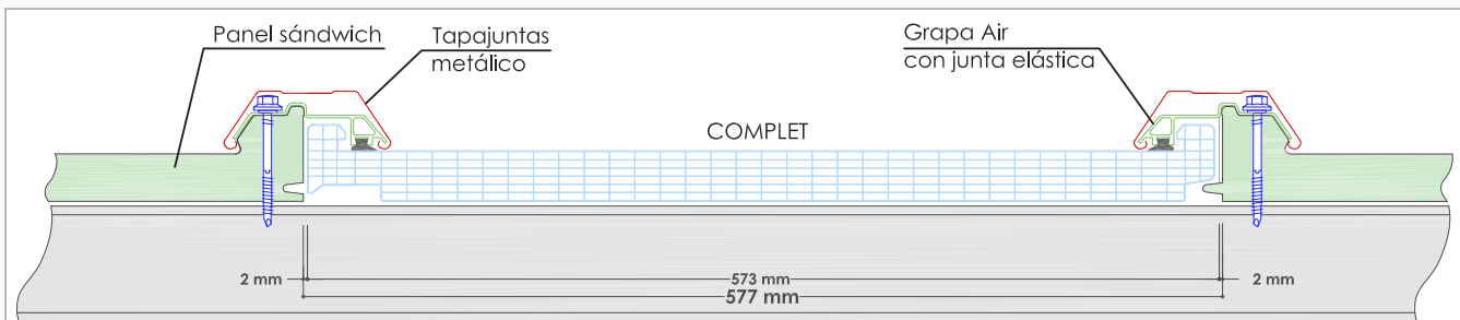
COLOCACIÓN PLACA SIMPLE
