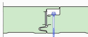
HI-PIR STX junta de panel
