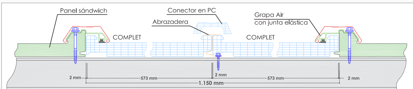
COLOCACIÓN PLACA DOBLE
